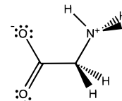
Glycine Zwitterion
